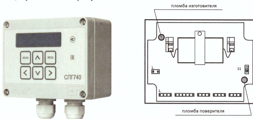
Рисунок 1 – Общий вид и схема пломбирования корректоров СПГ740
